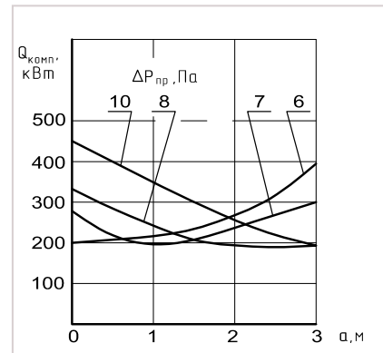
Рис. 3. Зависимость тепловой мощности компенсации от величины экранирования струи завесы
