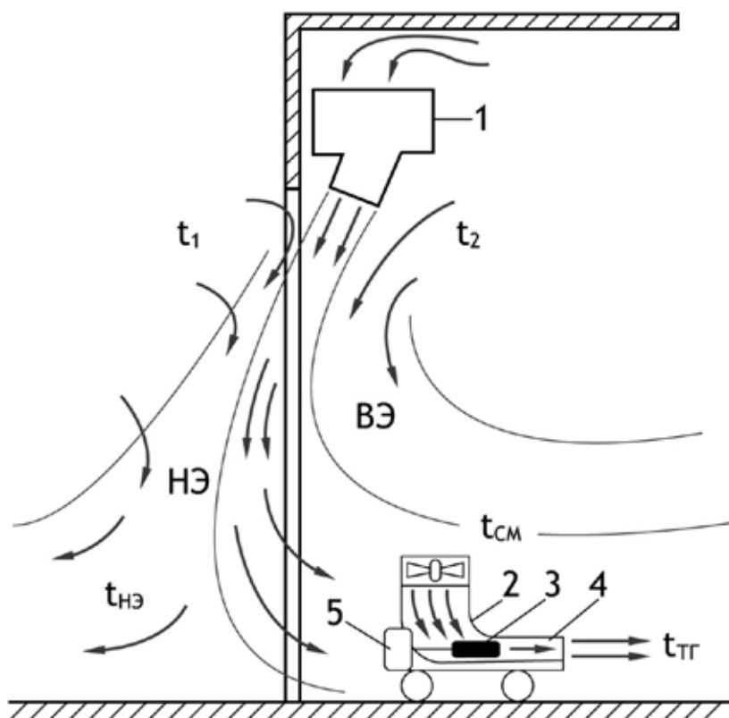
Рис. 1. Схема работы мобильного теплогенератора в проеме ангара
