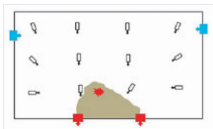
Рис. 8. Схема расположения поворотных струйных вентиляторов, ориентированных на очаг пожара, в помещении автостоянки
