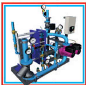
ТЕПЛОВЫЕ ПУНКТЫ
