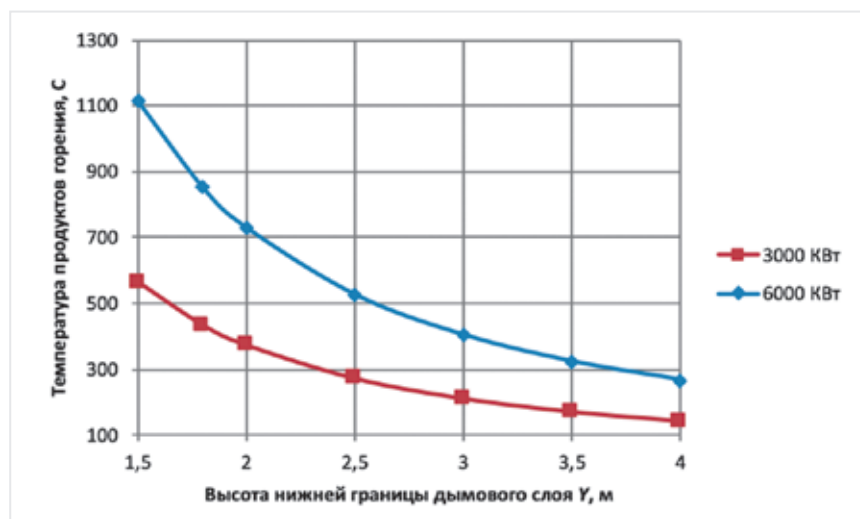
Рис. 1. График зависимости температуры продуктов горения t_{p2} от высоты нижней границы дымового слоя Y при пожаре автомобиля с двигателем внутреннего сгорания и электромобиля
