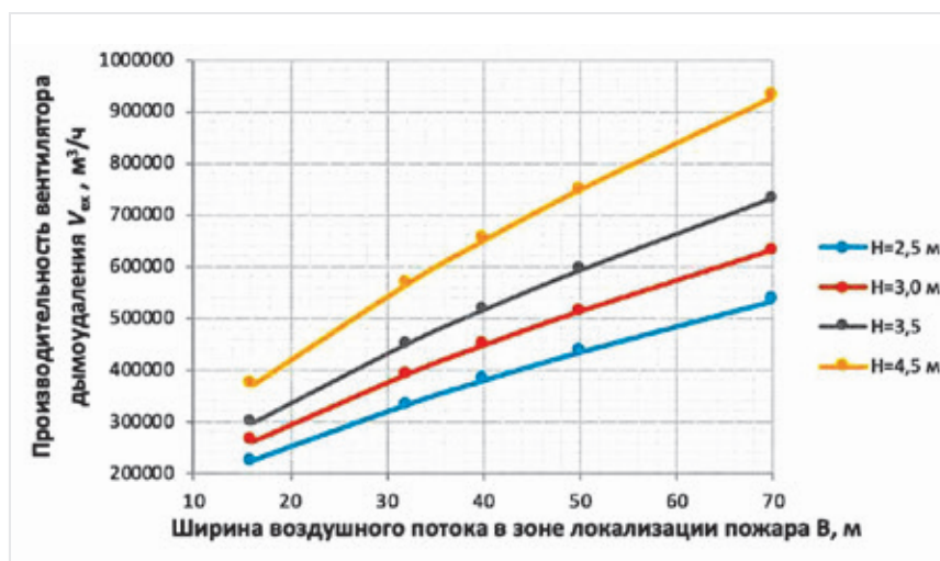
Рис. 3. График зависимости производительности вентилятора дымоудаления от ширины воздушного потока в зоне локализации очага горения электромобиля при различных высотах потолочного перекрытия при Q_K = 6000 кВт
