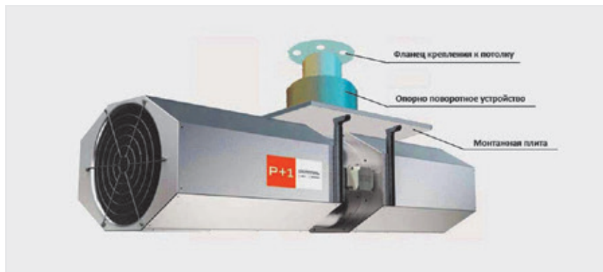
Рис. 7. Реверсивный струйный вентилятор с диаметром рабочего колеса 400 мм, с номинальной реактивной тягой 52Н, оснащенный опорно-поворотным устройством
